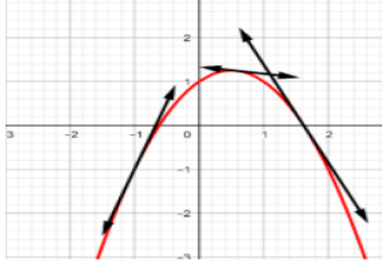
Graphique d'une fonction concave
